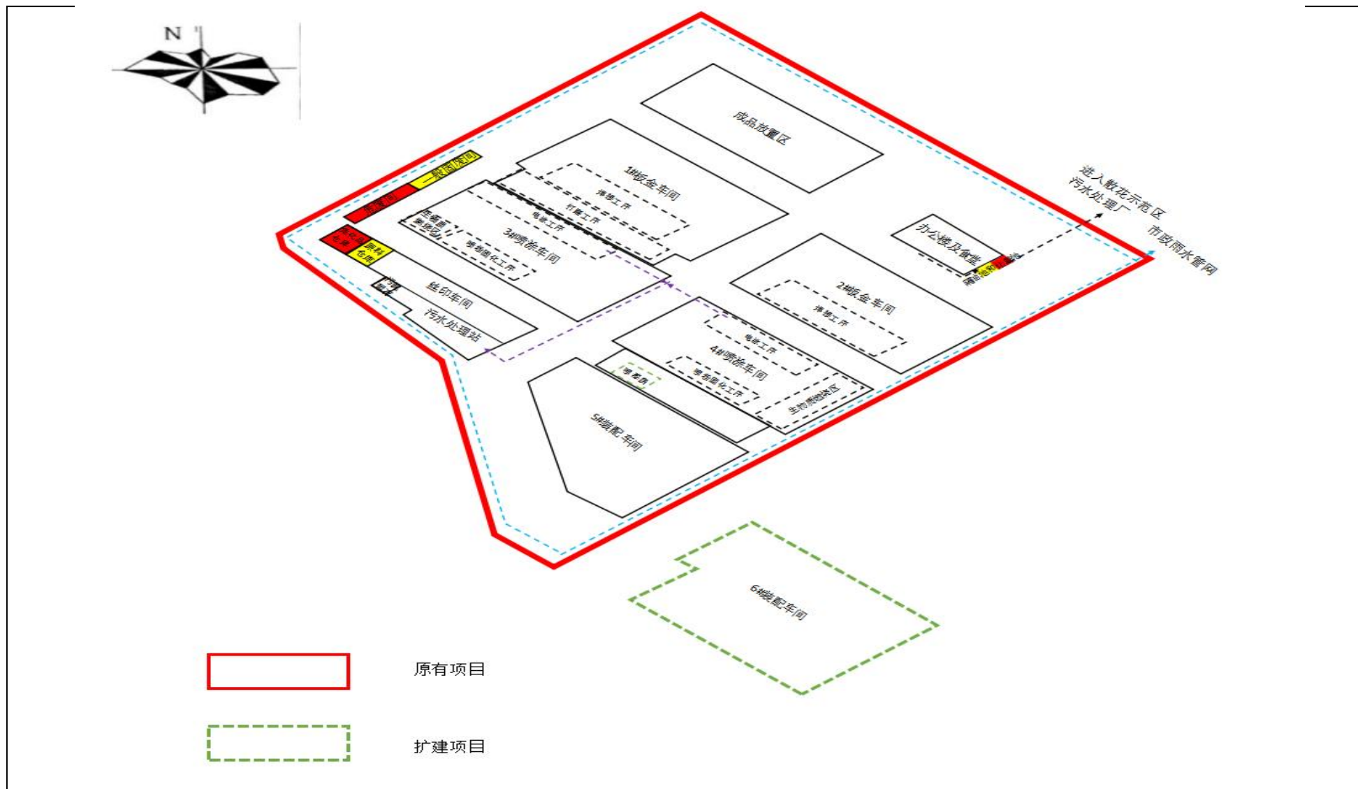
附图3 项目总平面布置图及雨污管网图
