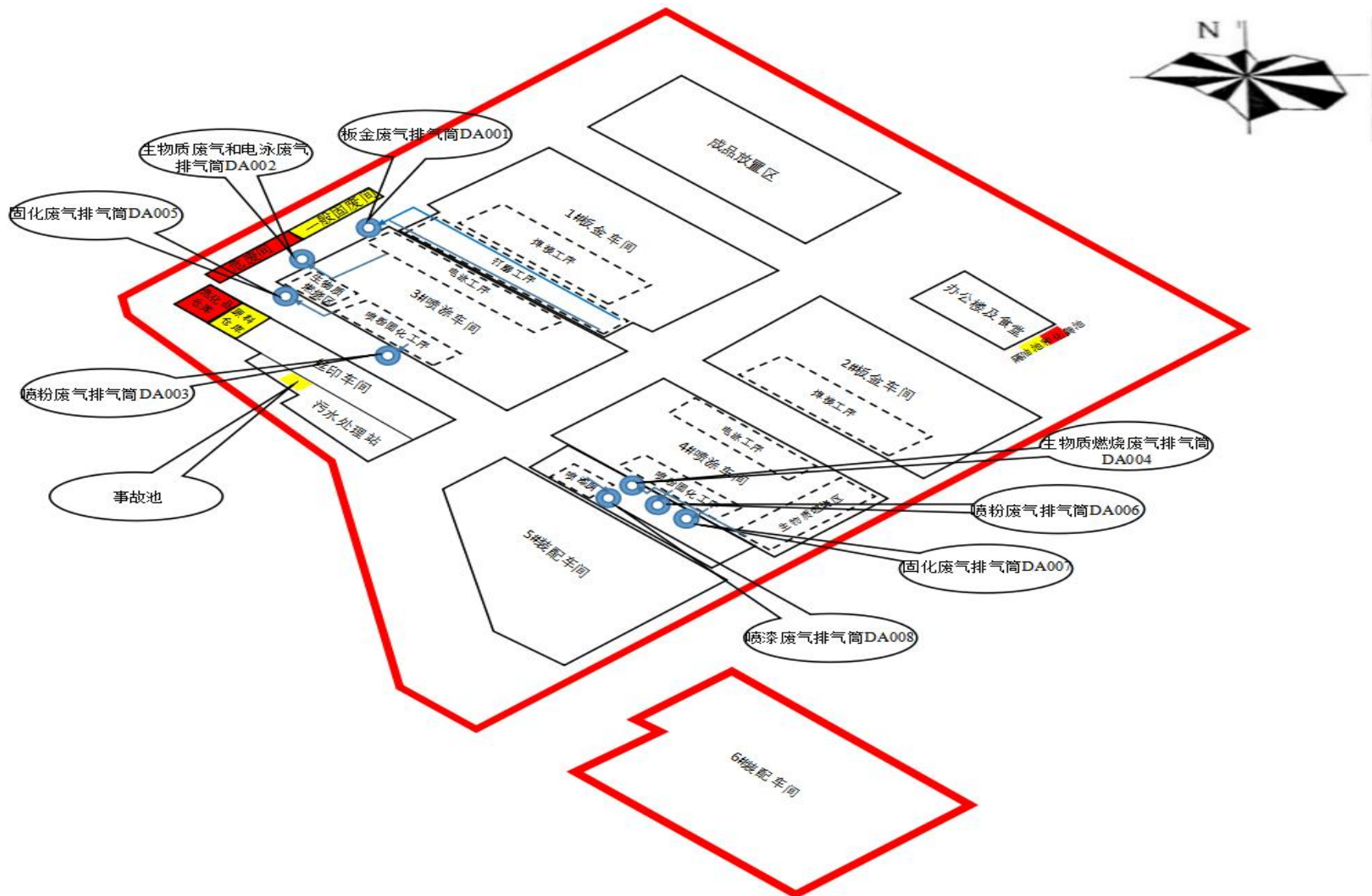
附图4 项目环保设施分布图
